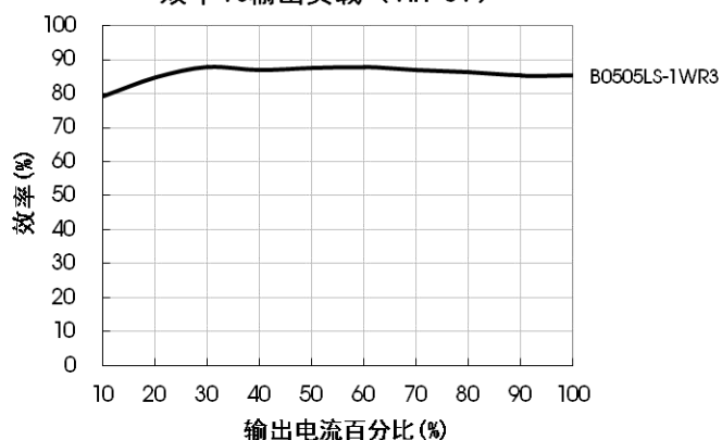
效率Vs输出负载 (Vin=5V)
